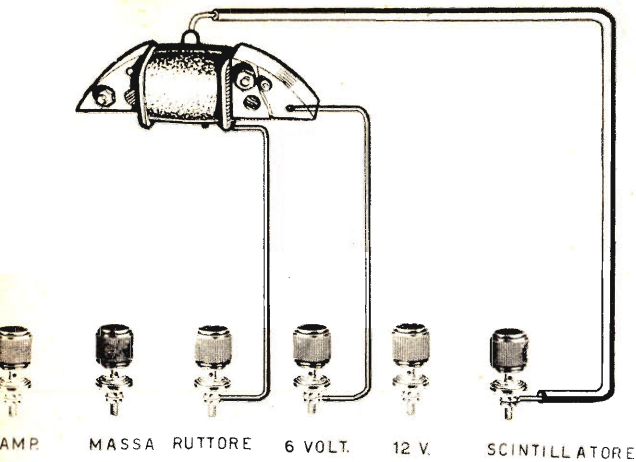
Fig. 3 - Per provare lo stato di una qualsiasi bobina d'alta tensione i collegamenti dovranno essere effettuati come in figura, prelevando la tensione di 6 oppure di 12 volt a seconda che la bobina appartenga al motore di una moto o di un'auto. Gli interruttori andranno regolati come è spiegato nell'articolo.
