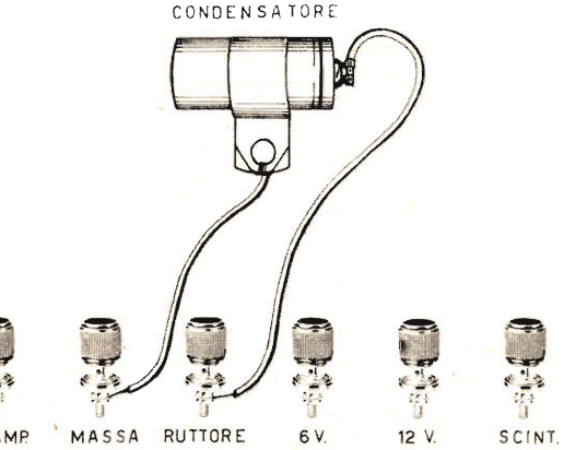
Fig. 3 - Per provare lo stato di una qualsiasi bobina d'alta tensione i collegamenti dovranno essere effettuati come in figura, prelevando la tensione di 6 oppure di 12 volt a seconda che la bobina appartenga al motore di una moto o di un'auto. Gli interruttori andranno regolati come è spiegato nell'articolo.
